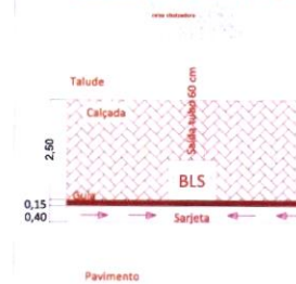
GUIA E SARJETA - Sem Escala (medidas em metro)
