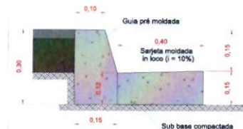
GUIA E SARJETA - Sem Escala (medidas em metro)
