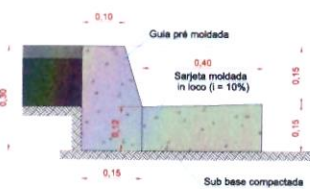
GUIA E SARJETA - Sem Escala (medidas em metro)
