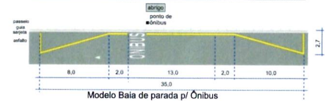
Modelo Baia de parada p/ Ônibus
