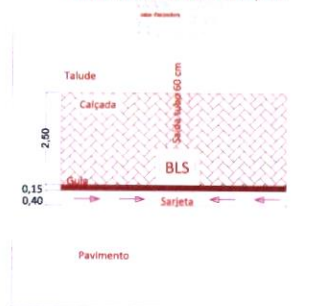
GUIA E SARJETA - Sem Escala (medidas em metro)
